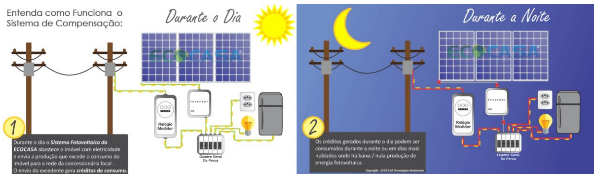
Figura 2. Sistema solar on-grid.
